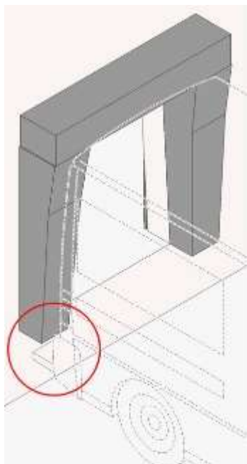
ASSA_ABLOY_Kissentorabdichtung_ohne_Bodenkissen
