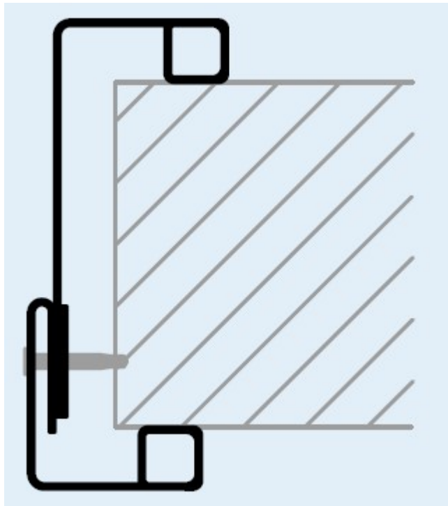
Umfassungszarge Helsiniki
