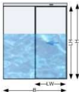
dokaLA stW1
