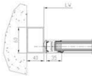
dokalA Anfahr 60_40
