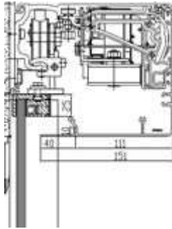
dokaIA Glasklemmschiene
