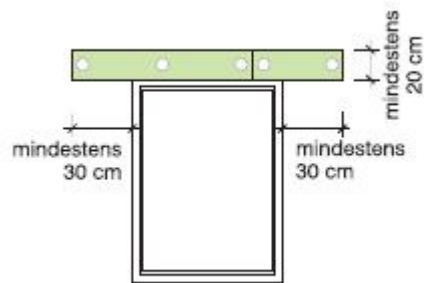
SYN_Brandschutzriegel
