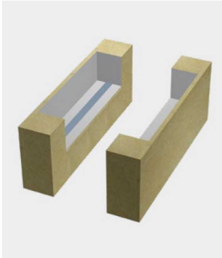
Capatect Schürzenelement MW plus Schürze aus MW mit 3-seitiger Aufdoppelung, und Montageschiene
