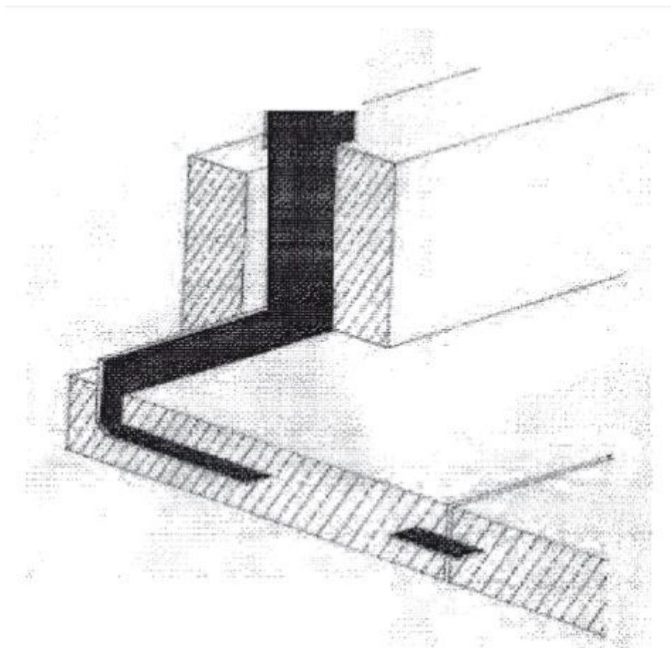
Fugendichtblech
