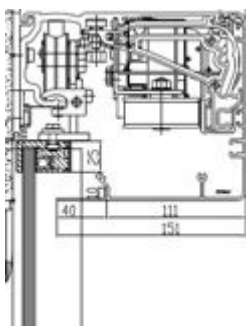
dokaIA Glasklemmschiene
