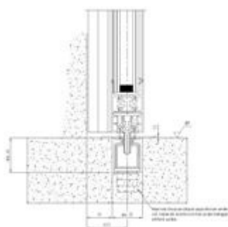
dokalA Bodenschiene
