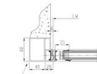
Mindest-Auflage auf Seitenwand = 35mm dokalA Anfahr60_6s
